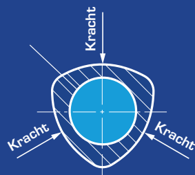
De klemdiameter wordt rond
